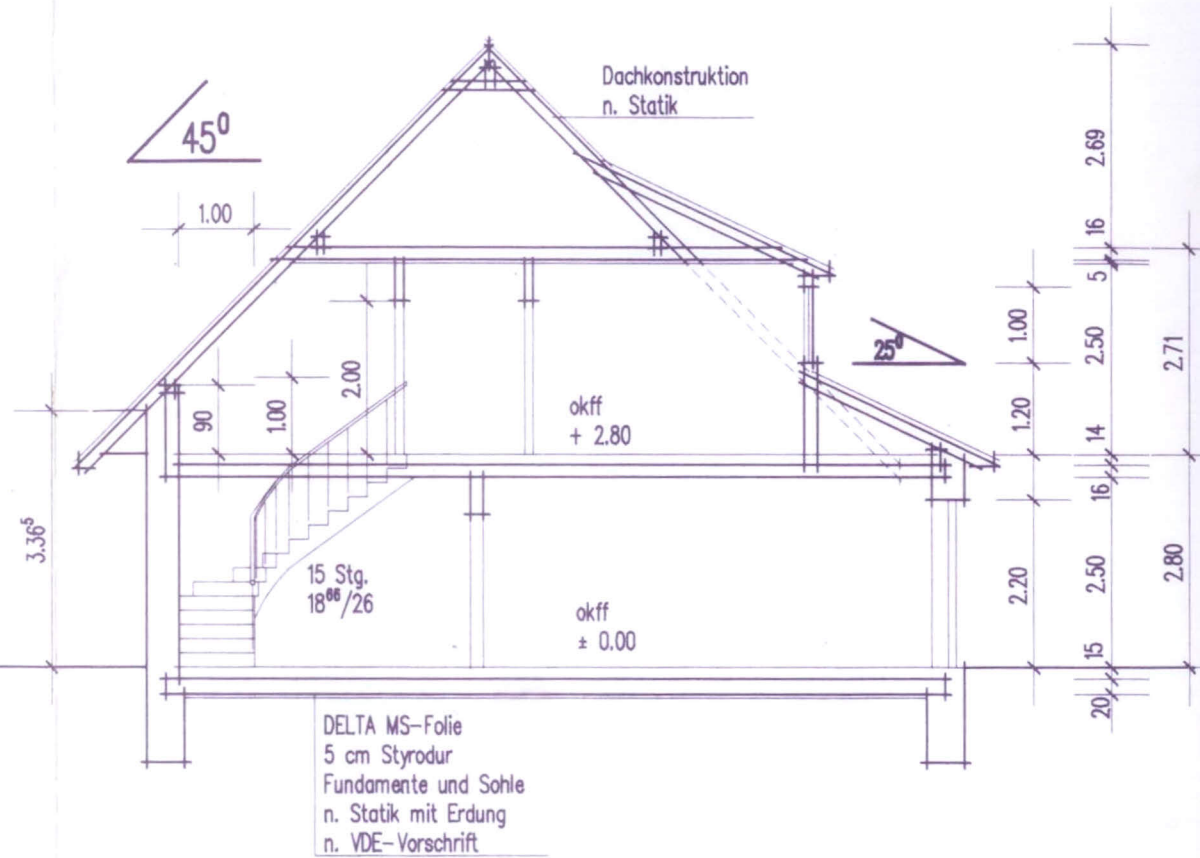
Schnitt
